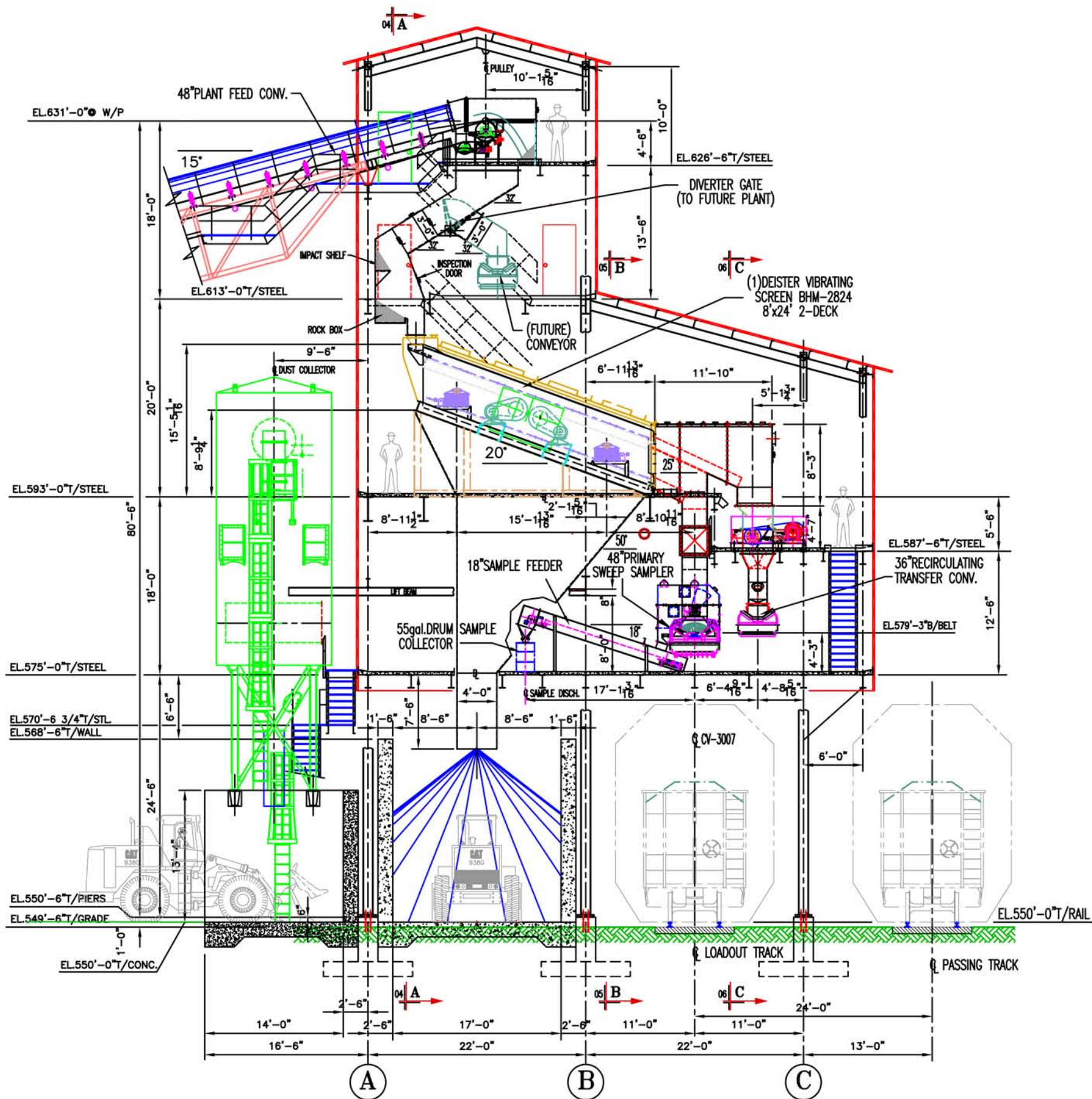
SECTION D-D
